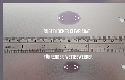
OBERFLÄCHENAUSBREITUNG (Drei Tropfen auf Stahloberfläche nach 5 Minuten)
